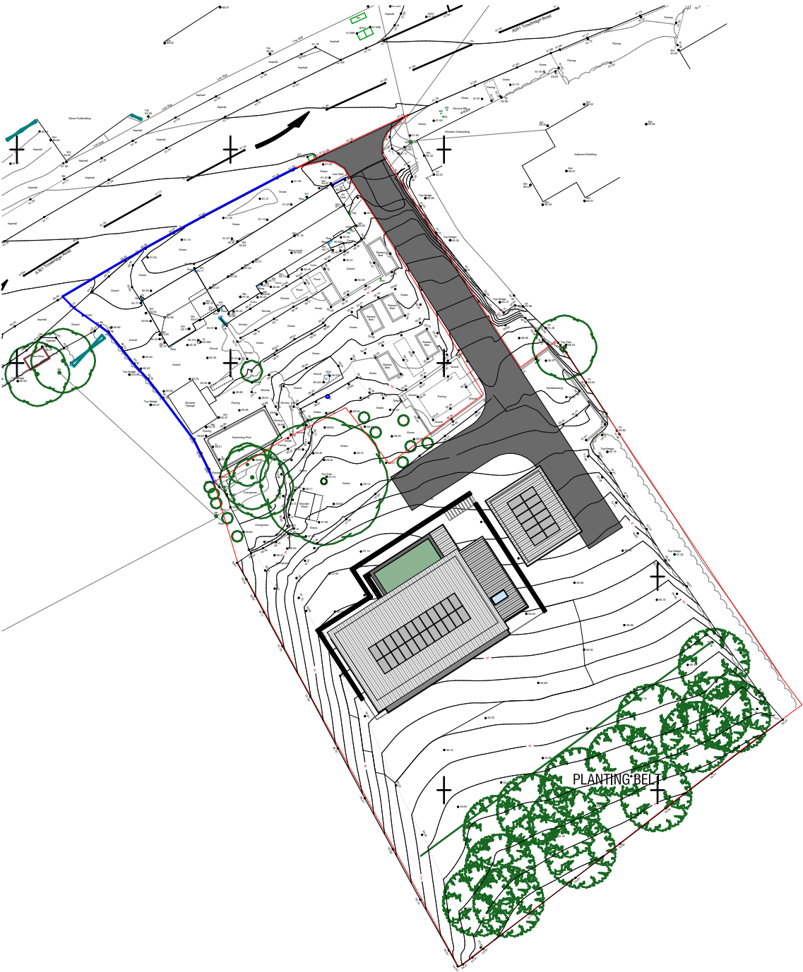
SITE PLAN 1:500
