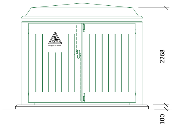
Elevation - A
