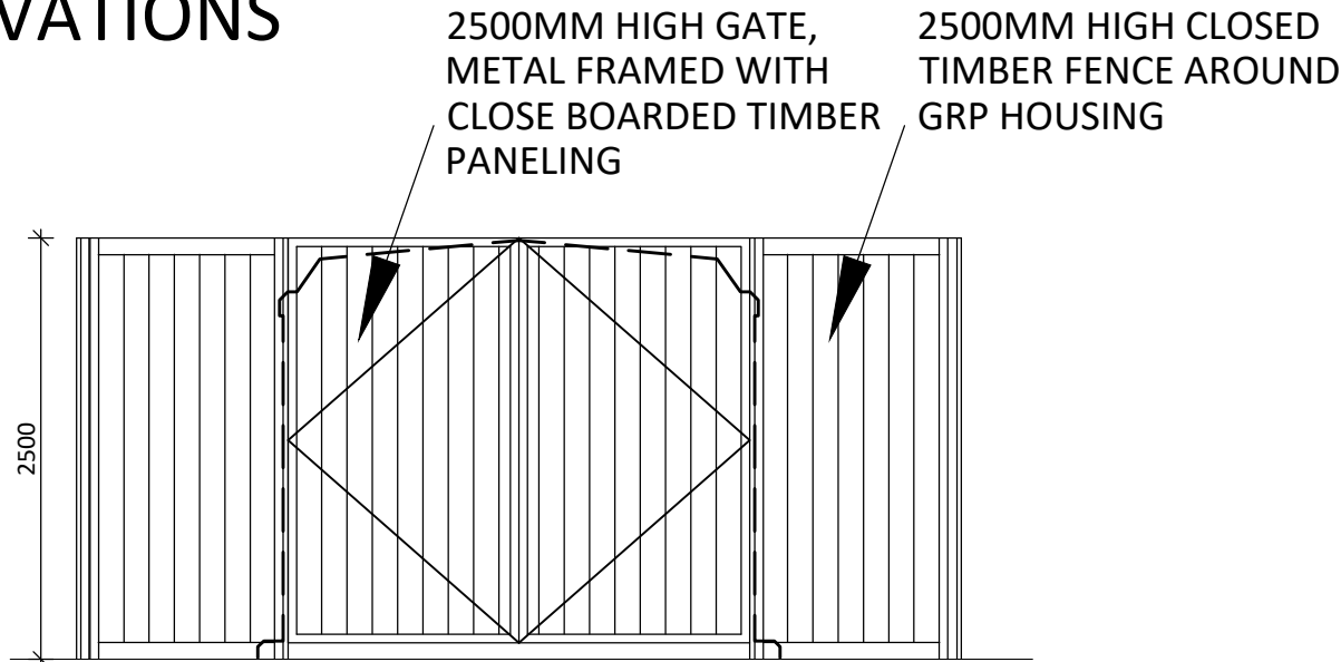
Elevation - A
