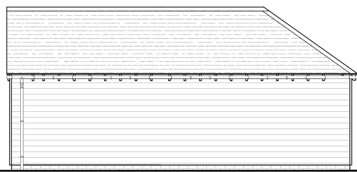
SW ELEVATION 1:100
