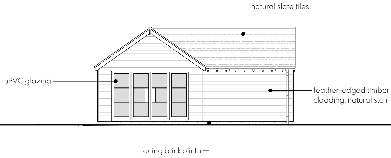
NE ELEVATION 1:100
