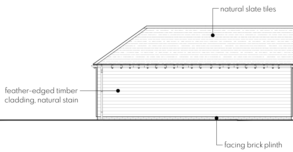
SE ELEVATION 1:100
