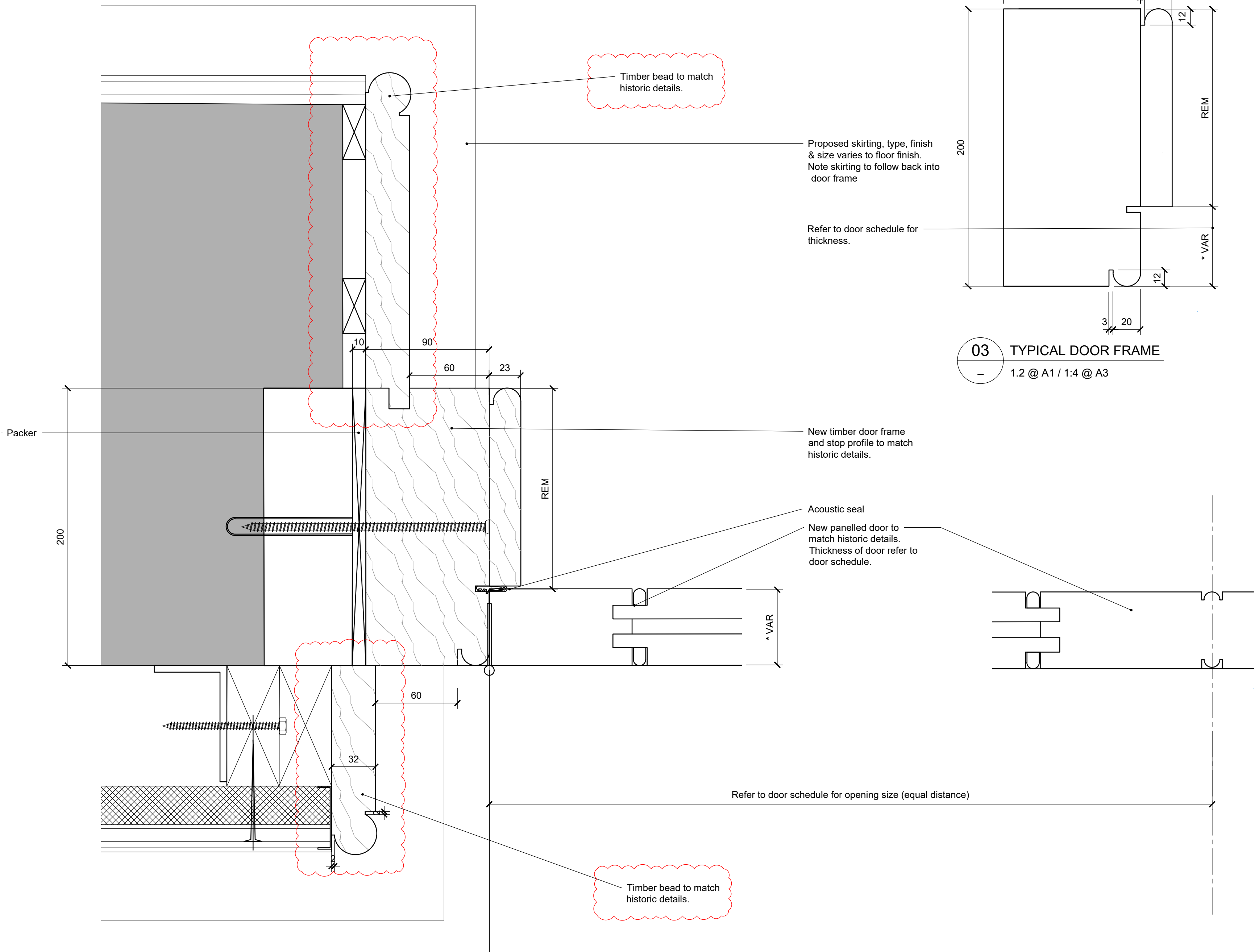
02 JAMB DETAIL 222 1.2 @ A1 / 1:4 @ A3
