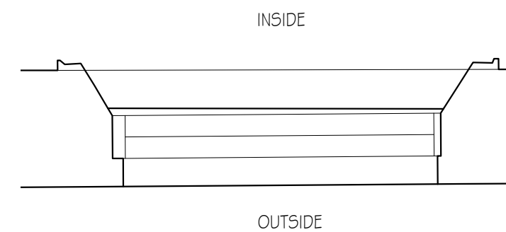
WF06 PLAN 1:20
