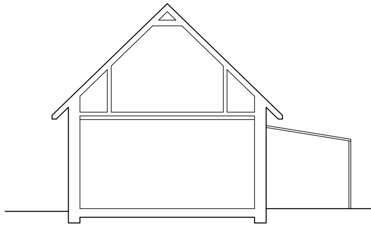
SECTION A-A
