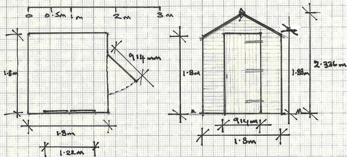
ELEVATION N
