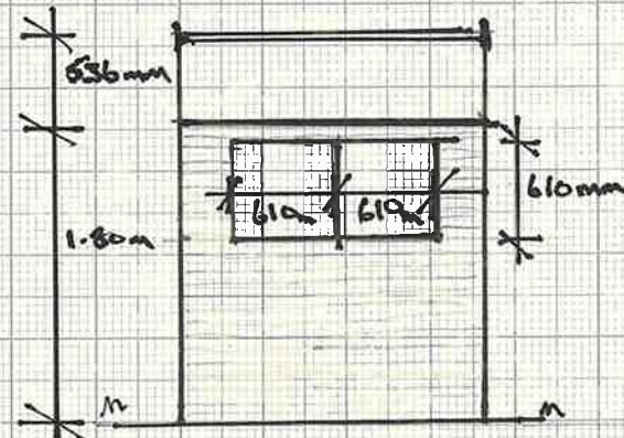
ELEVATION E
