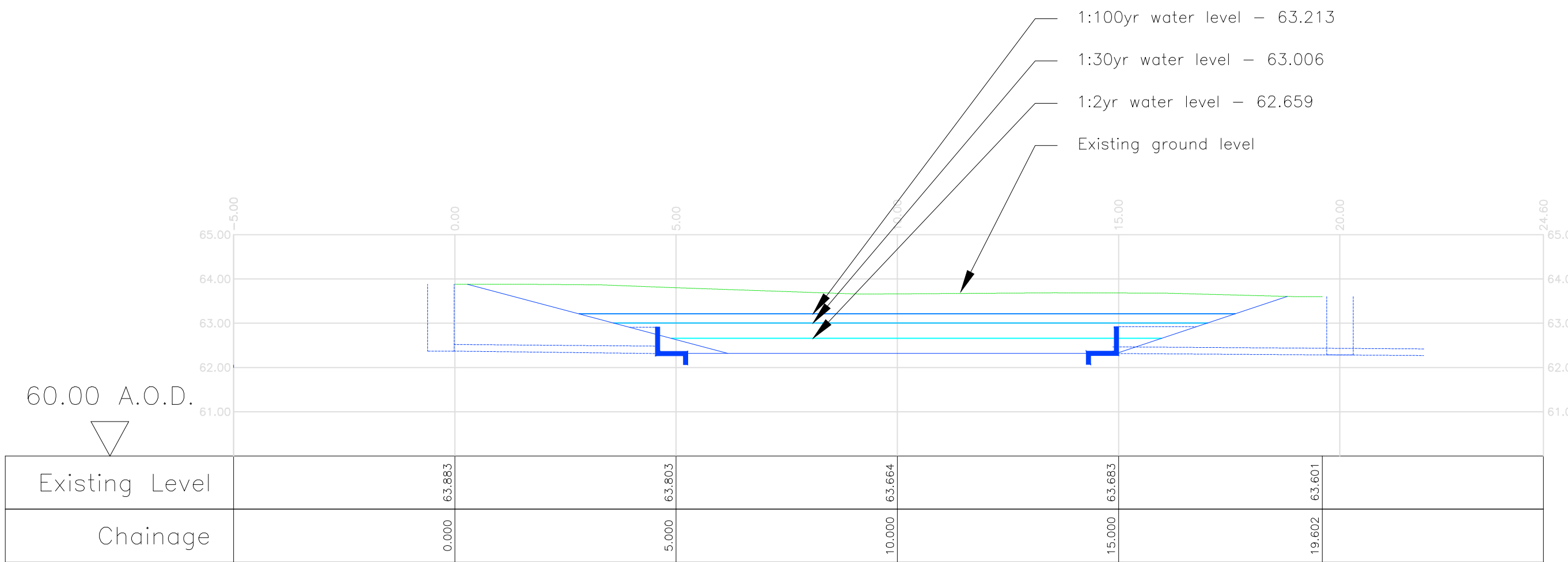
Horiz. 1:100 Vert. 1:100
