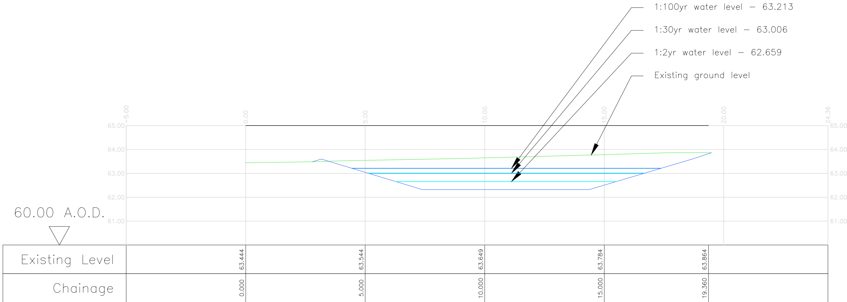
Horiz. 1:100 Vert. 1:100
