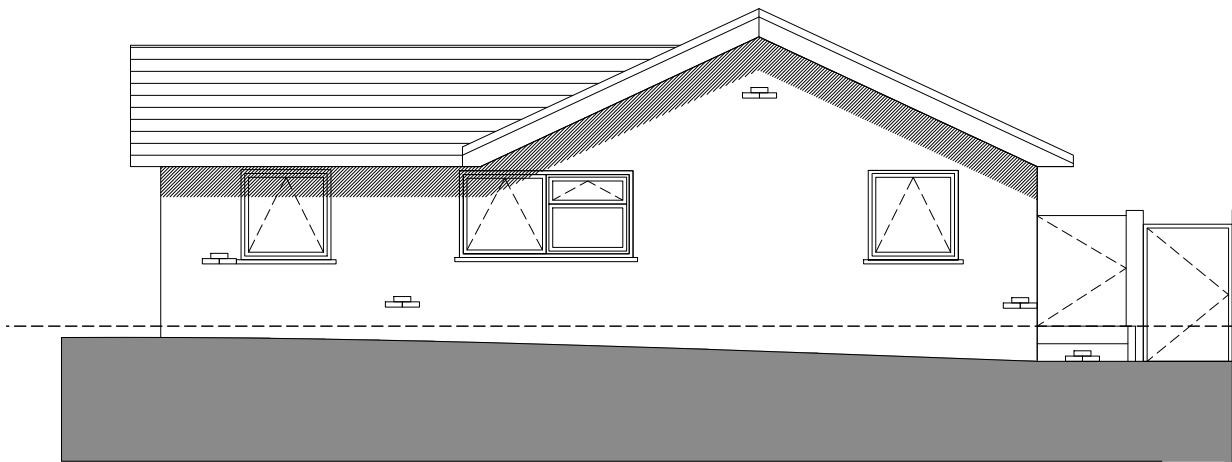
Elevation 01 1:100
