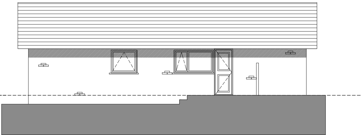
Elevation 04 1:100
