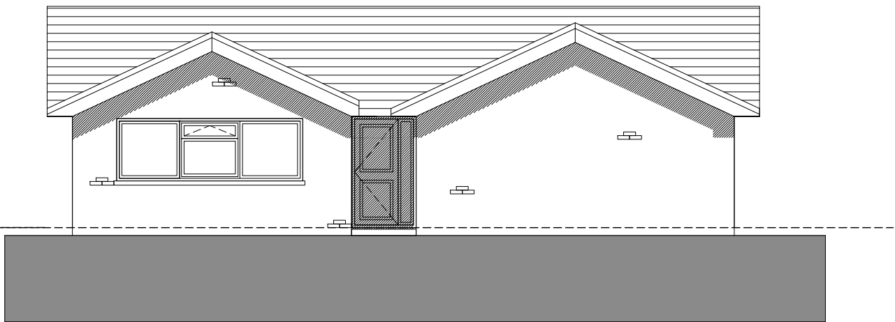
Elevation 02 1:100
