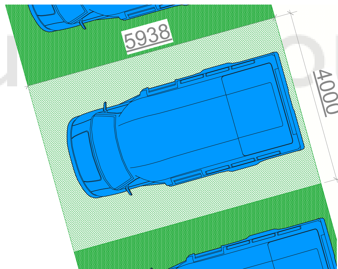
6 Mini Bus x 5 Scale: 1:50
