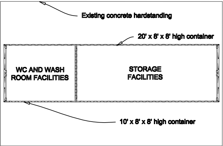
Plan 1:100
