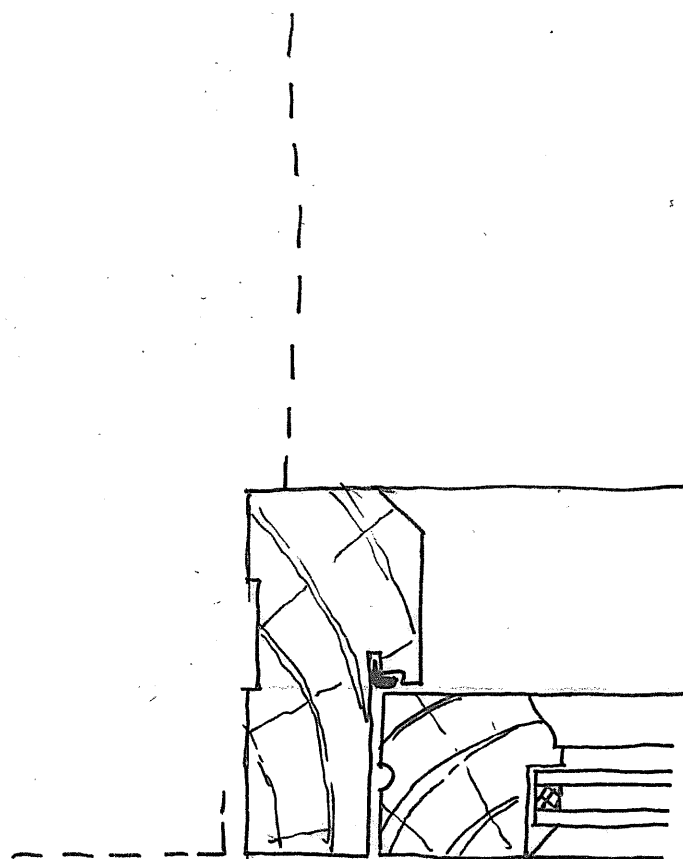
JAMB DETAIL
