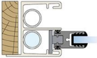
Jamb detail upper sash
