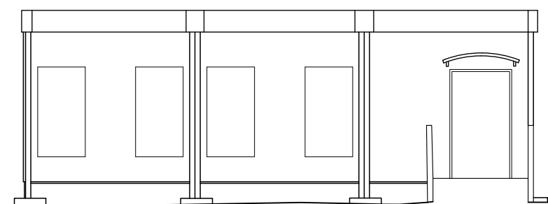
ELEVATION 10
