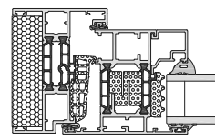
➤ 58BW FLUSH HI JAMB
