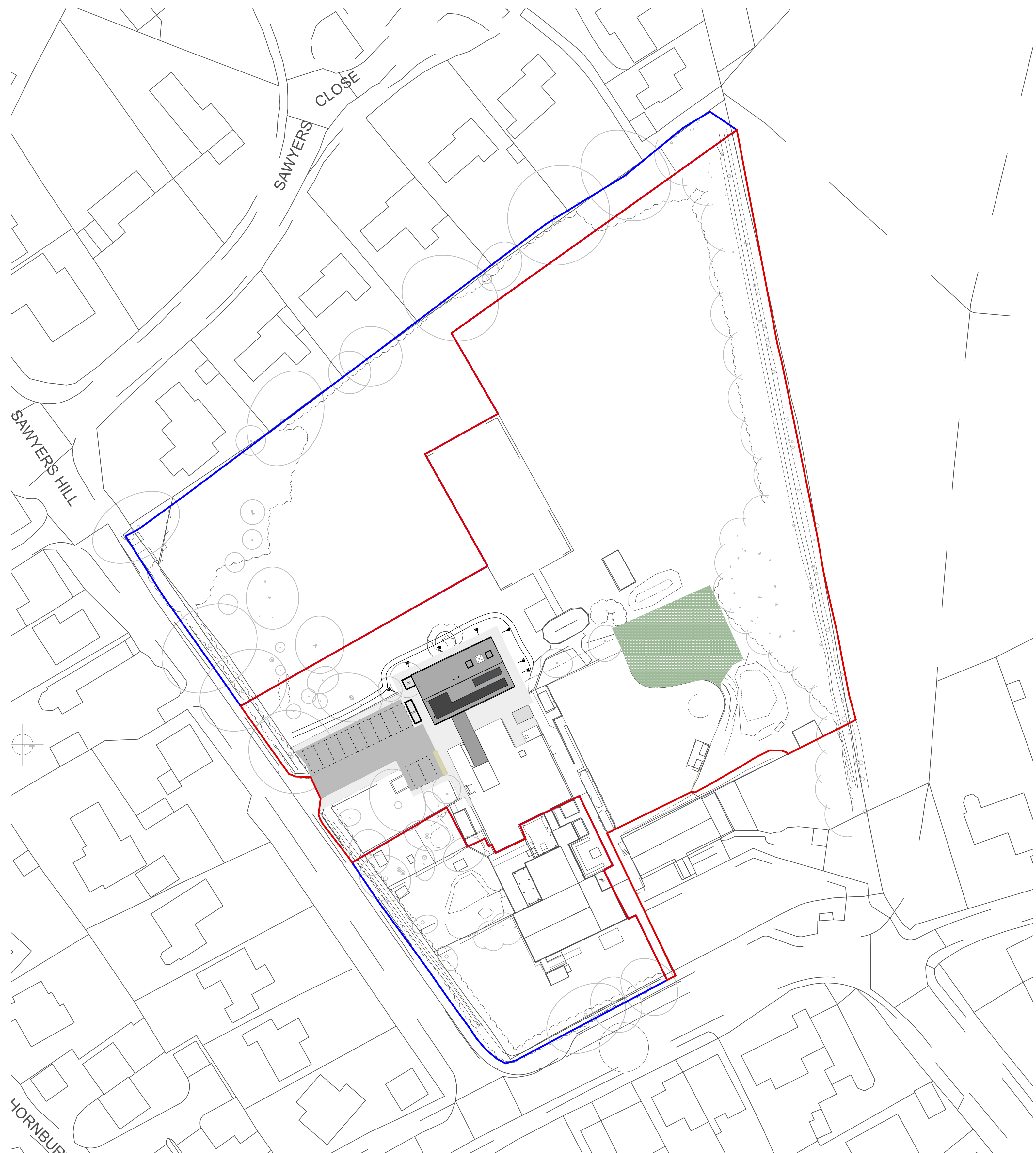
2 Block Plan Scale: 1:500
