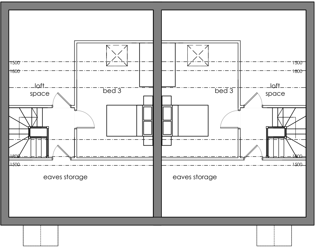
Loft Plan
