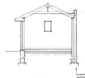
Section A-A 1-50
