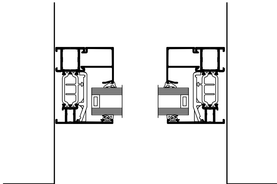
1:2 Jamb Detail
