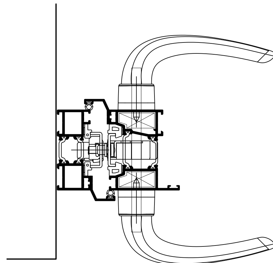
1:2 Jamb Detail
