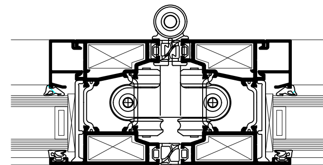
1:2 Folding sliding door detail
