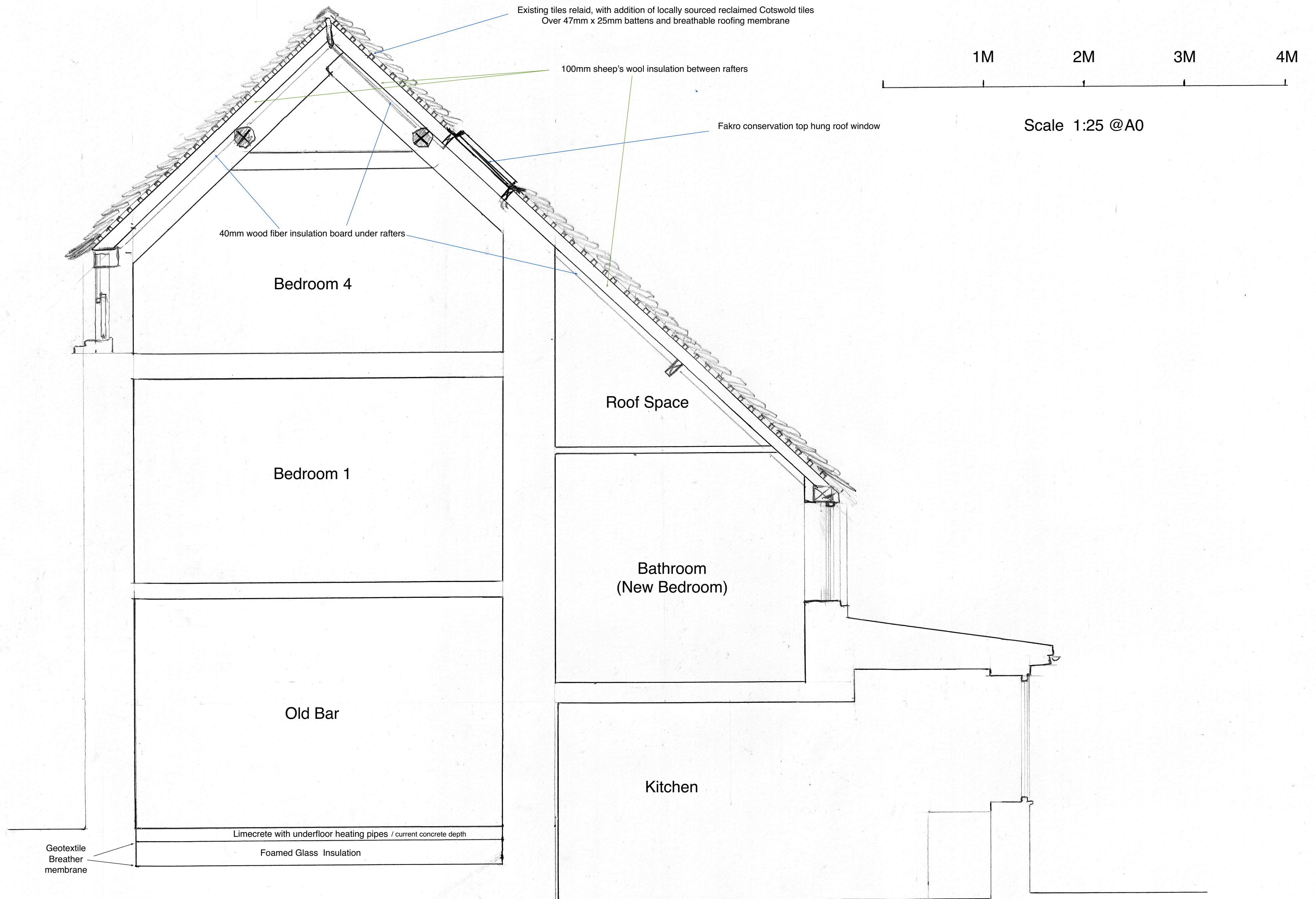
SECTION A-A
