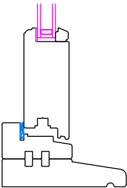
Door Cill
