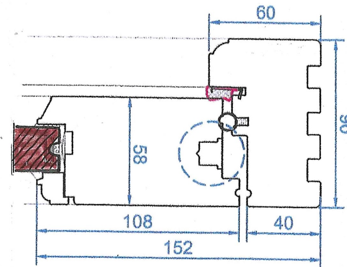
Jamb
