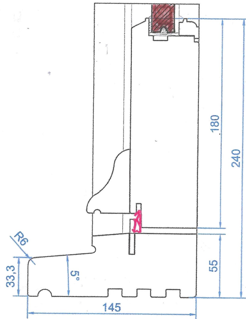
Cill
