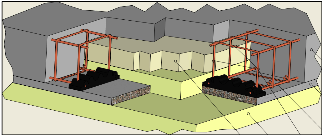
DETAIL B SCALA 1/5 DETALLE B ESCALA 1/5
