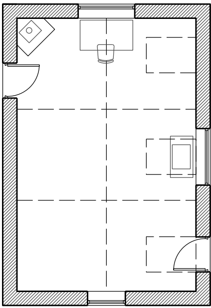
FF PLAN 1:100
