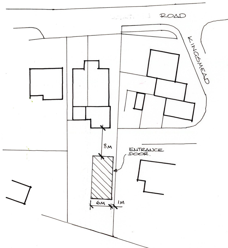
SITE PLAN 1:500
