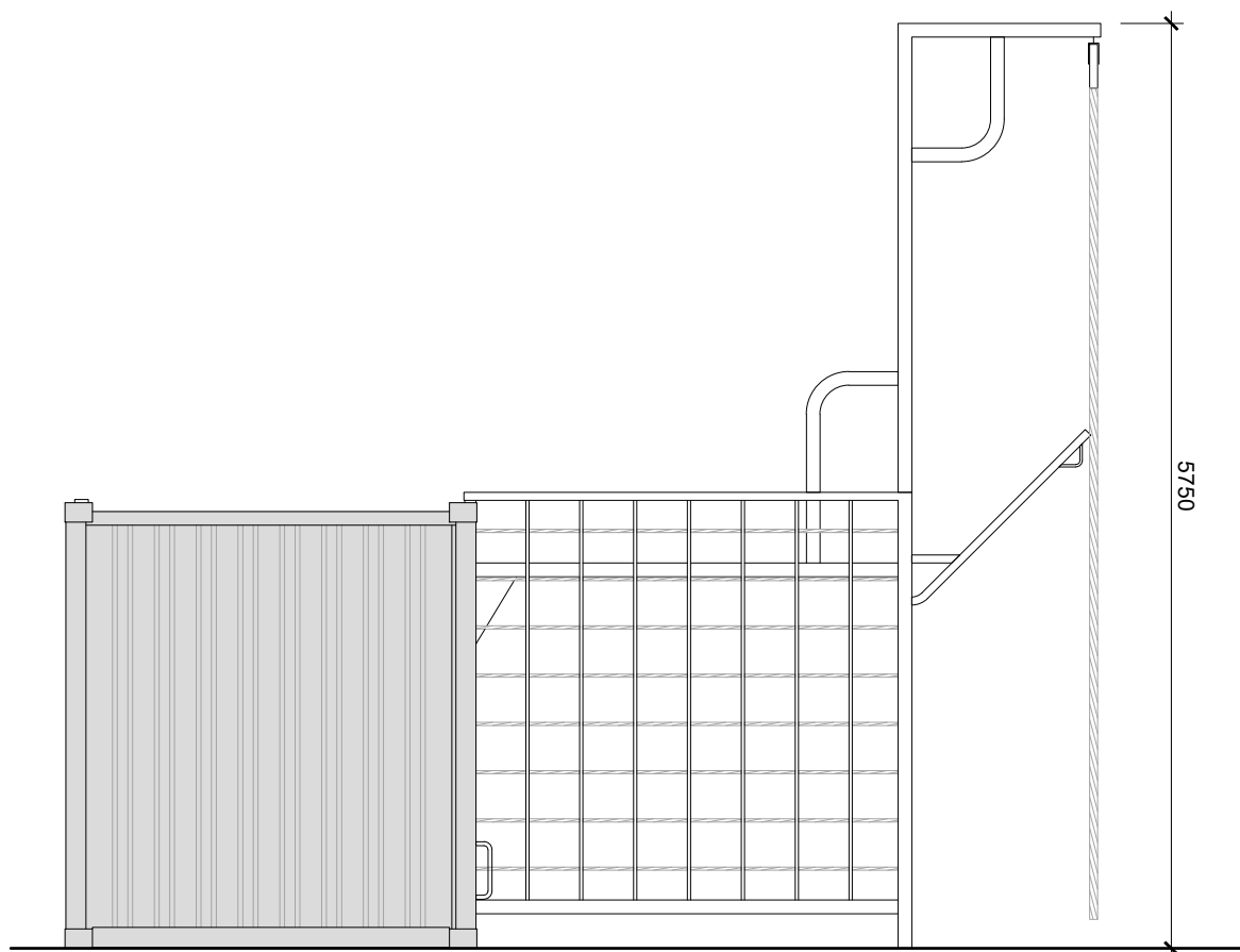
ELEVATION 01
