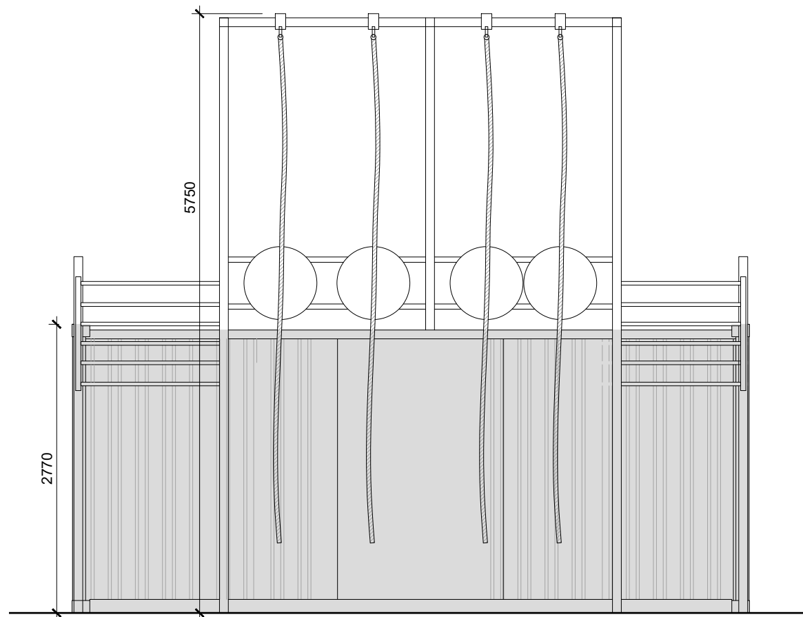
ELEVATION 04
