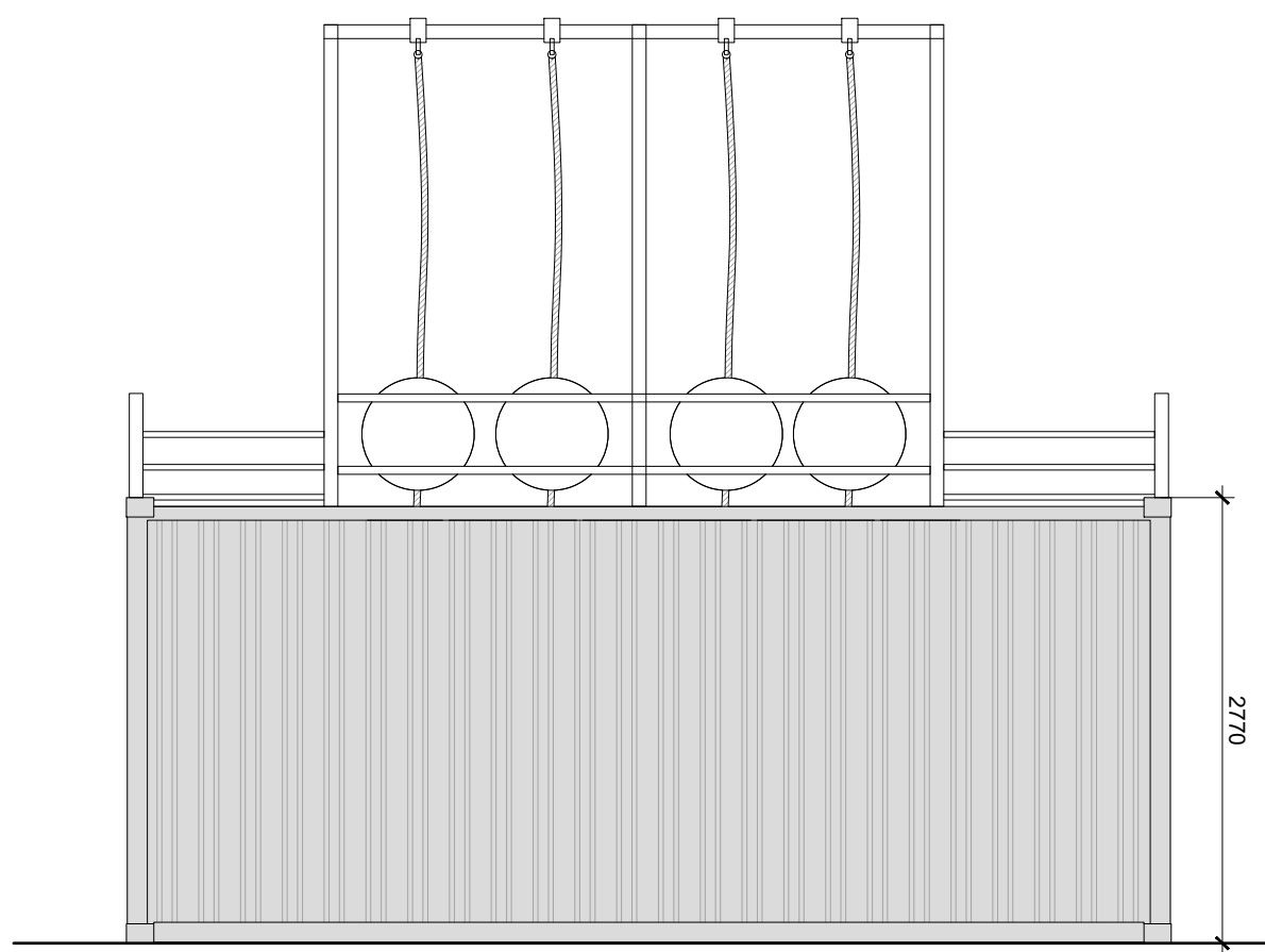
ELEVATION 02
