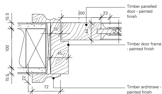
07 Door plan detail - 1:5
