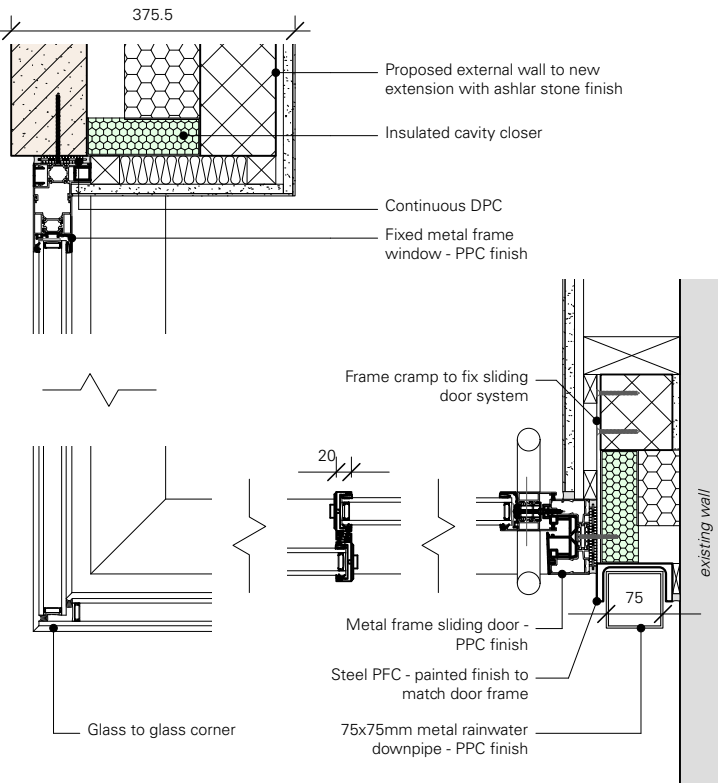
04 Door / Window jamb details - 1:10
