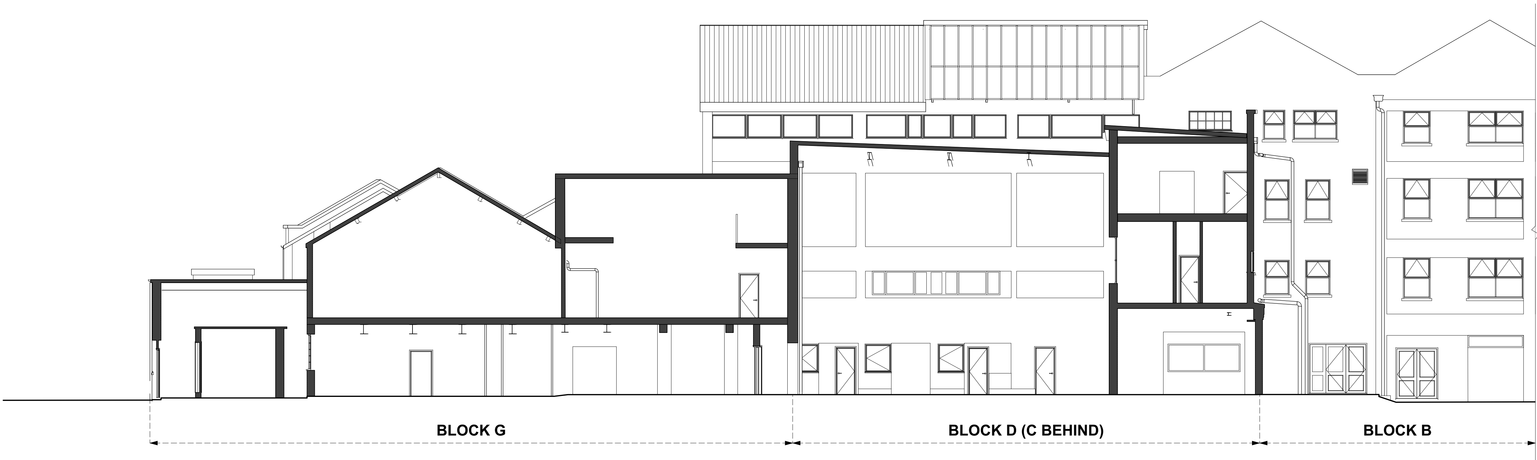
1 Existing Section AA Scale: 1:100
