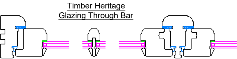
Window Typ. Jamb
