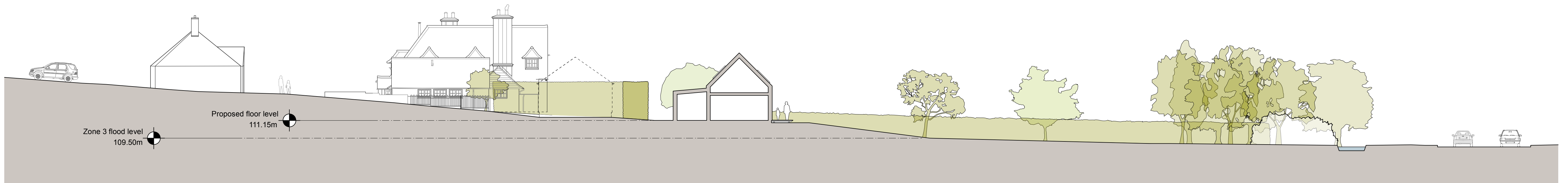
Long Section BB 1:200
