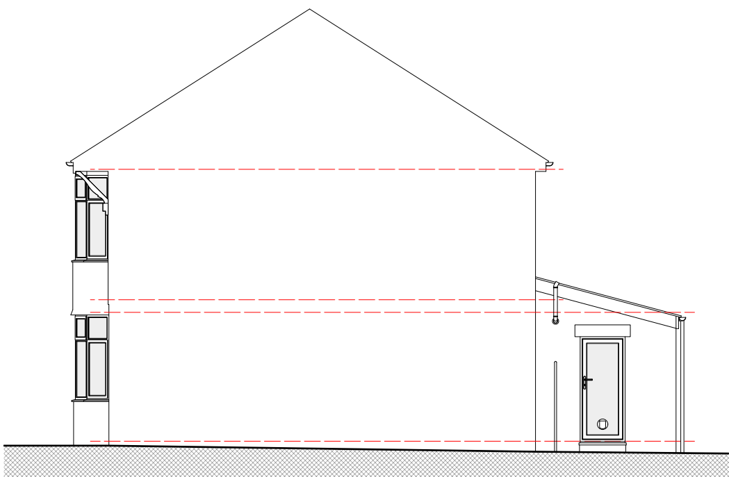
ELV 04 Existing E Elevation 1:100
