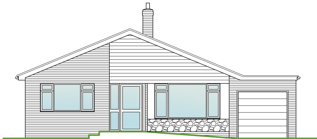
Existing SE Elevation
