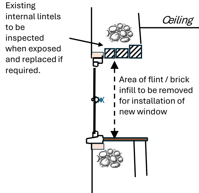
Section A – A (Scale: 1.20 @ A4)
