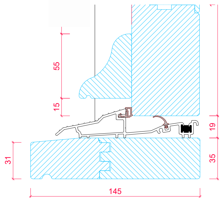
DOOR DEX 1 & 2 - SECTION SCALE 1:2
