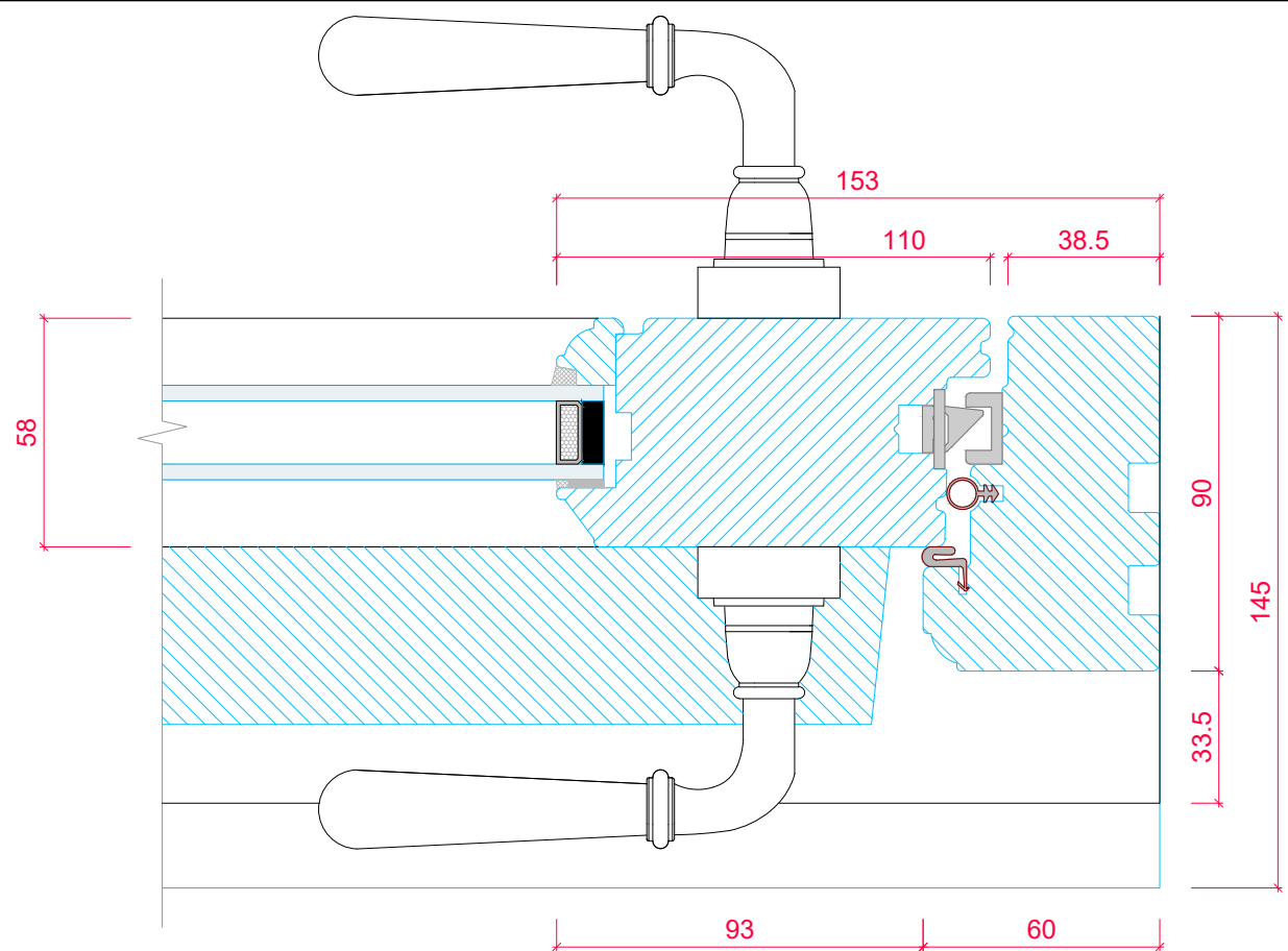
DOOR DEX 1 & 2 - PLAN SCALE 1:2
