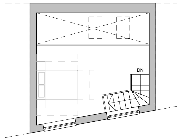
2 Level 1 1 : 100
