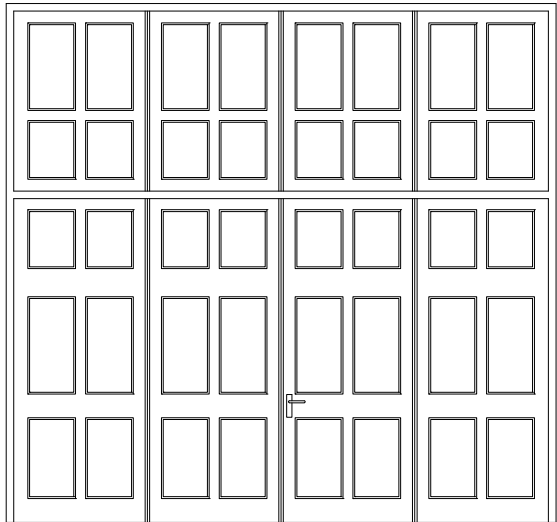
A-A DOOR ELEVATION
