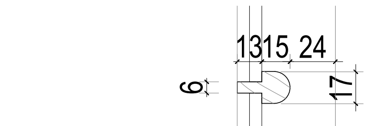
7. Section 1:20
