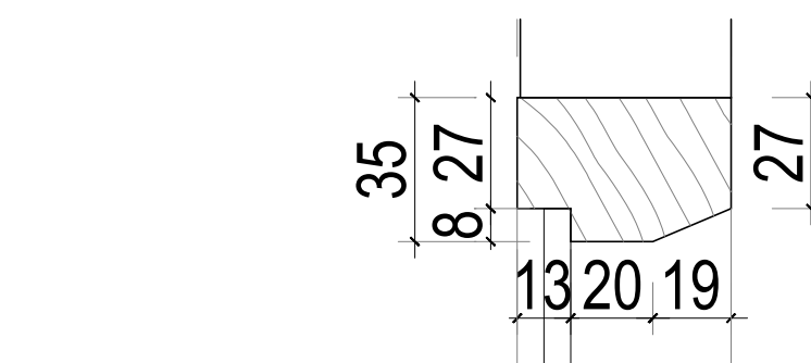
6. Section 1:20
