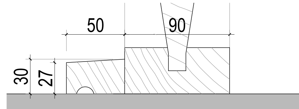
10. Section 1:20
