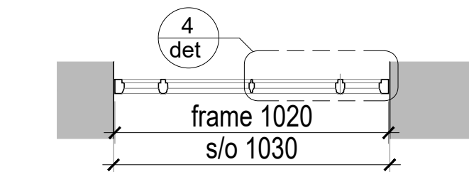
2. Plan 1:20
