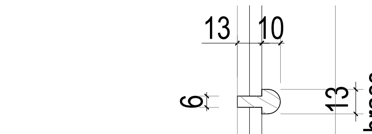
8. Section 1:20
