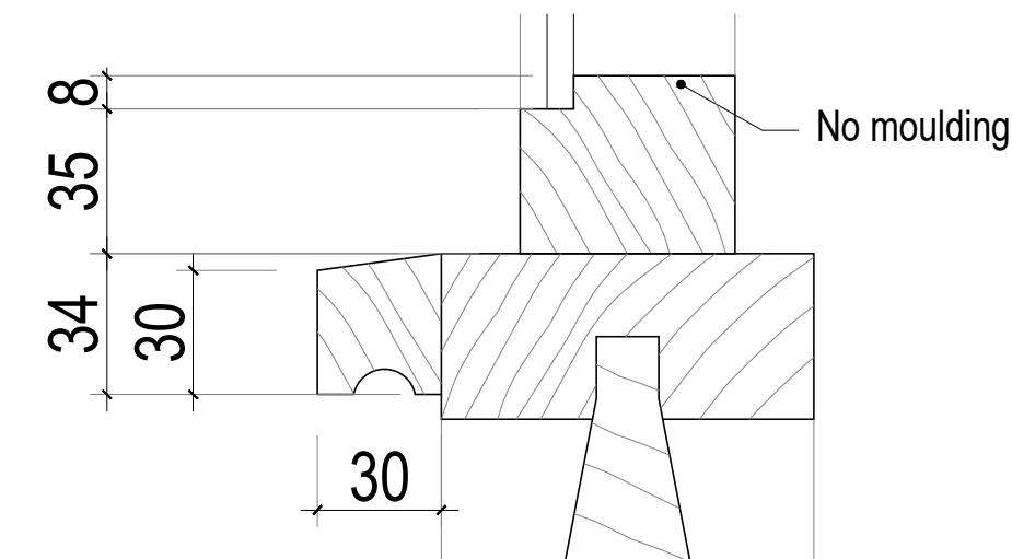
9. Section 1:20
