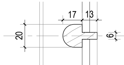
6. Section 1:5
