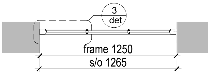
2. Plan 1:20
