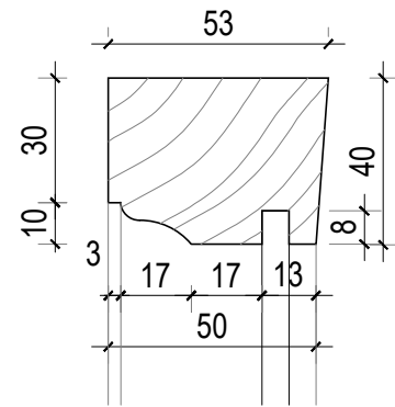
5. Section 1:5
