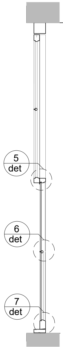
4. Section 1:5
