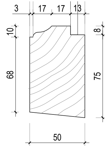
7. Section 1:5
