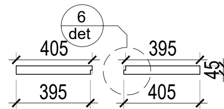
4. Plan 1:20
