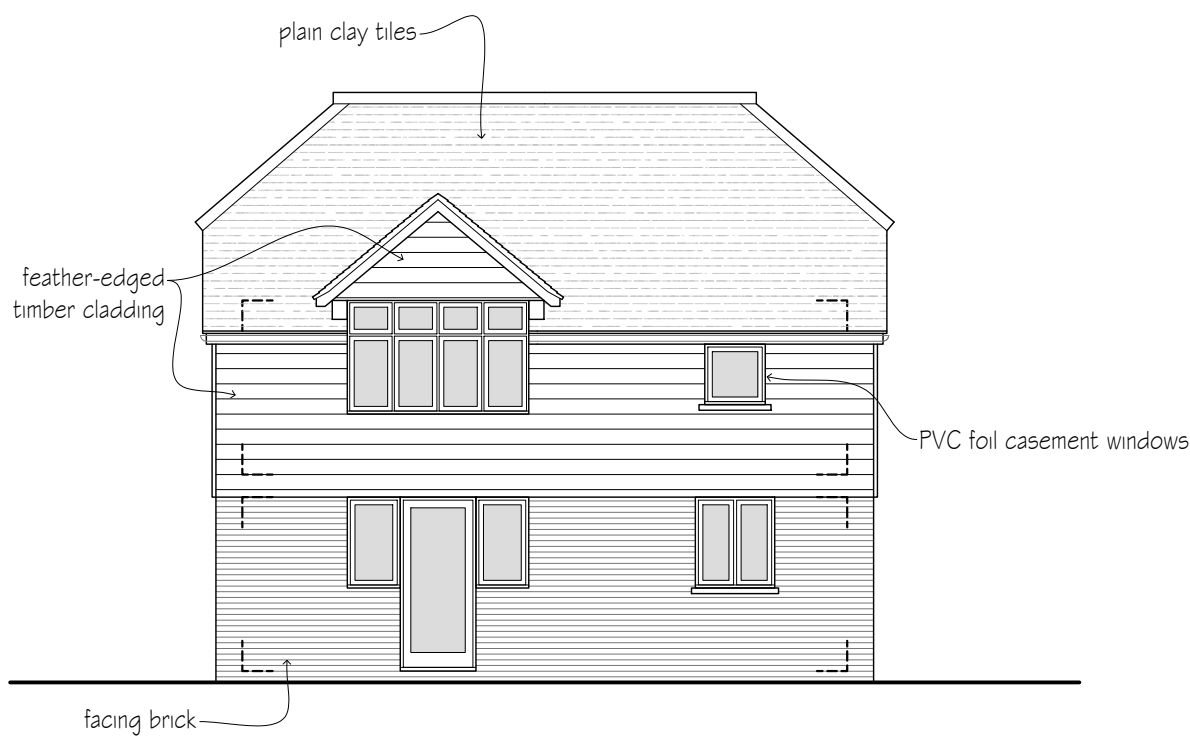
SE ELEVATION Plot 3
