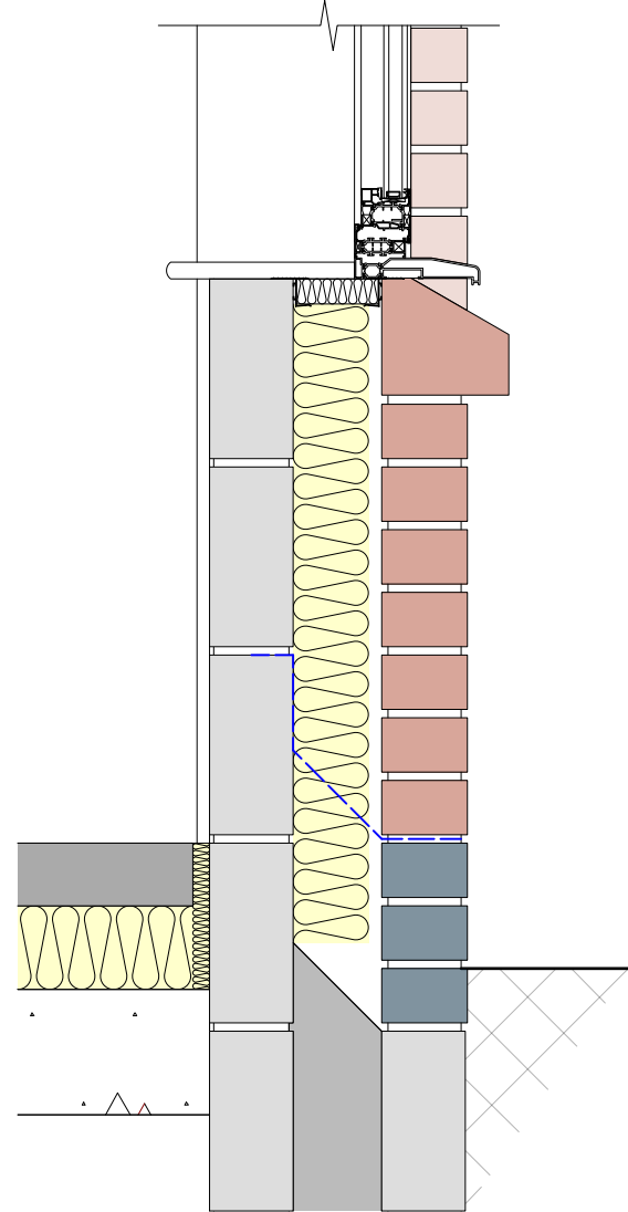
DET 07 Windowcill 01 1:10
