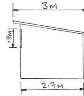
END ELEVATION
