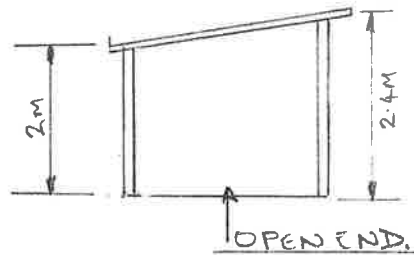
END ELEVATION
