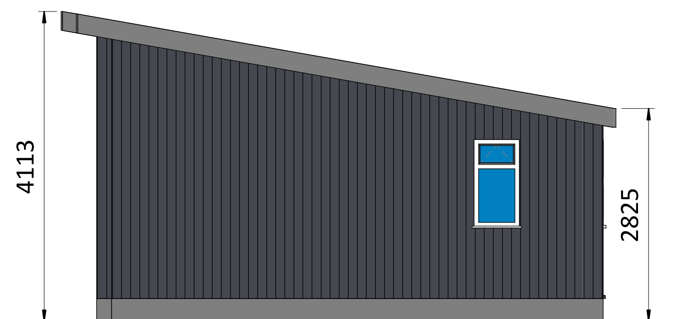
3 End Elevation (En suite double bedroom)
