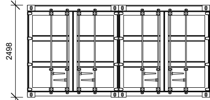
EXG. FRONT ELEV 1:100
