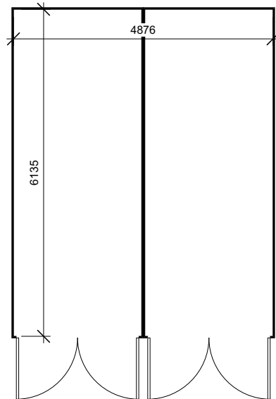
EXG. PLAN 1:100
