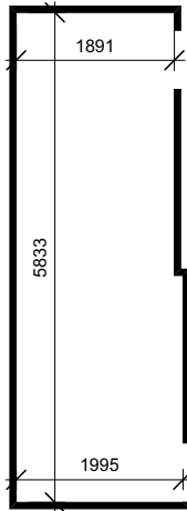
EXG. PLAN 1:100
