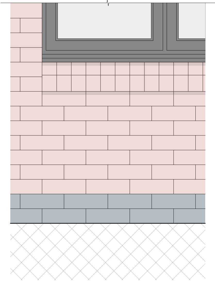
DET 08 Windowcill 02 1:10
