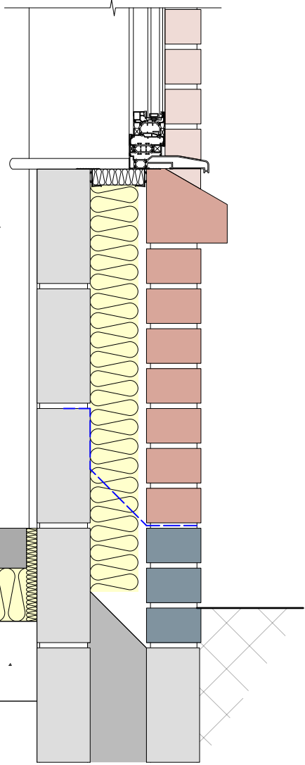
DET 07 Windowcill 01 1:10
