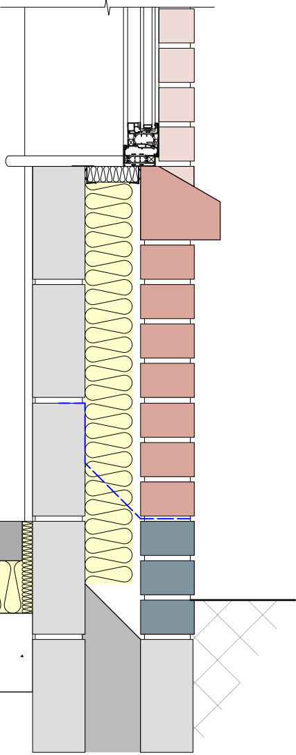
DET 08 Windowcill 02 1:10
